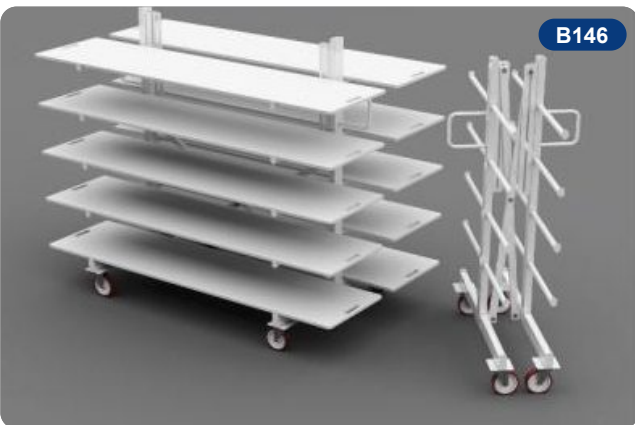
رف راحة القماش (وجهين) Double Sided Fabric Resting Racks عرض 120 × طول 200 × ارتفاع 180 سم
