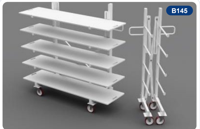
رف راحة القماش (وجه واحد) Single Sided Fabric Resting Racks عرض 60 × طول 200 × ارتفاع 180 سم
