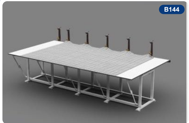
تراييزة فرد قماش بدبابيس قابلة للإمالة (أي مقاس) Tilting Pin Table for Fabric Spreading
