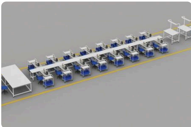
تخطيط خط إنتاج كامل (خياطة وكي وتجهيز) Complete production line layout
