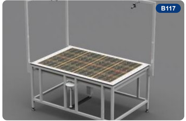
تراييزة دبابيس قابلة للضبط بالليزر Adjustable Pin-Table with Laser عرض 120 × طول 180 × ارتفاع 85 سم
